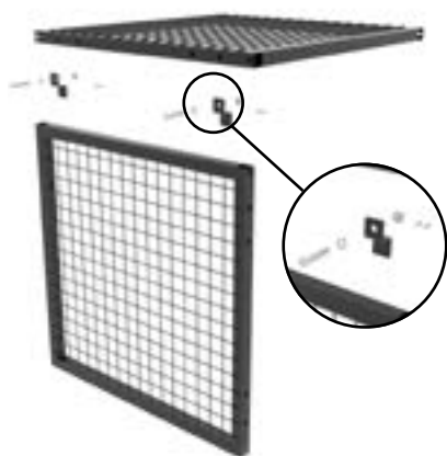
07 KIT CONEXIÓN TECHO
